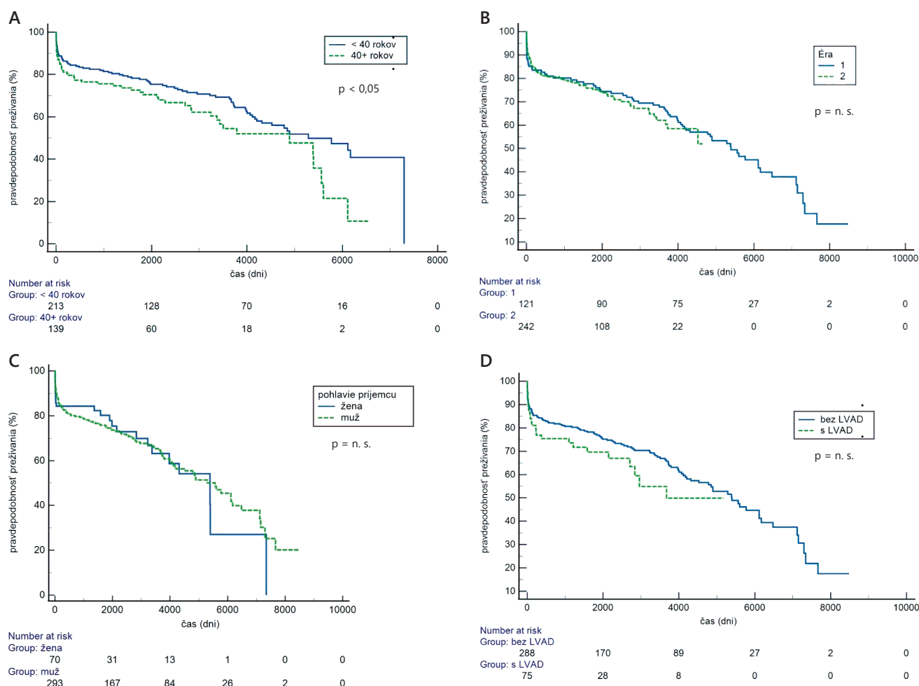
Obrázok 2 Kaplan-Meierova krivka prežívania pacientov po HTx v závislosti od: A – vekovej skupiny darcu (vek darcu < 40 rokov verus \geq 40 rokov); B – éry, v ktorej podstúpili transplantáciu (Éra 1 = < 2008, Éra 2 = 2009 – 2021); C – pohlavia príjemcu; D – implantovanej mechanickej podpory ľavej komory (LVAD) pred transplantáciou (MP = mechanická podpora)
